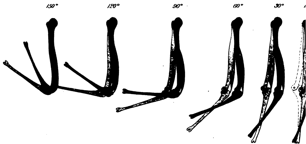
Anfang der Streckbewegung des unbelasteten Arms bei alleiniger Contraction eines eingelenkigen Streckmuskels des Ellbogengelenks für verschiedene Ausgangsstellungen.
